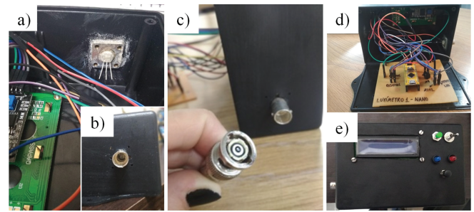
Figura 3: a) Fixação do TSL237s-LF junto a um conector BNC fêmea na caixa Patola®; b) visão exterior da conexão do TSL237s-LF; c) fibra óptica com o conector BNC macho para fácil acoplamento da sonda de medição; d) circuito e conexões internas do luxímetro finalizado; e) exterior do luxímetro finalizado.
